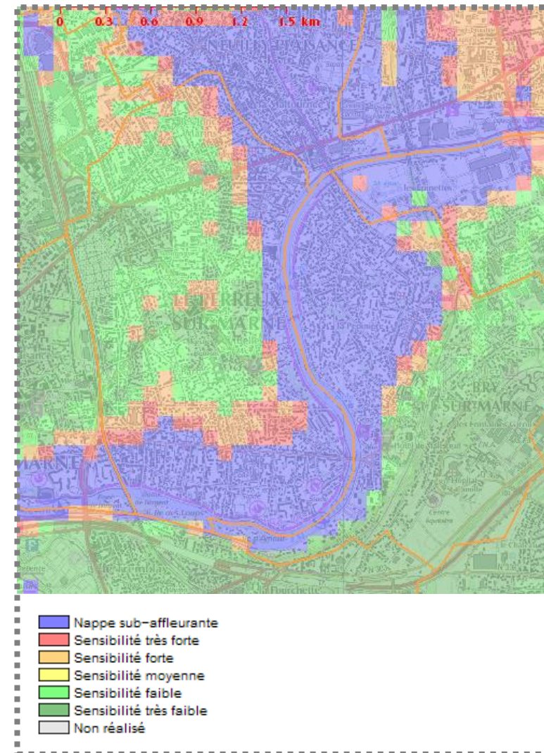
Aléa inondation par remontée de nappe
